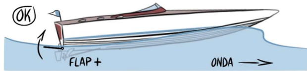
Pag. 91 , utilizzo dei flap nell'assetto trasversale (sopra) e utilizzo dei flap con onda a favore (a destra)
